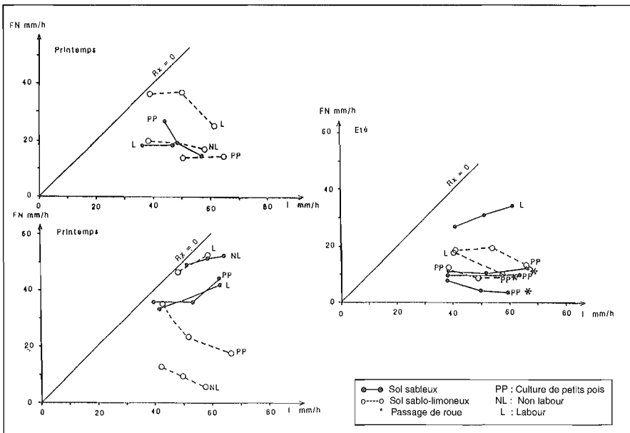
Figure 6 : Relations FN = f(I) pour deux campagnes de mesure et pour différents états de surface de sols du site du Val d'Orléans (d'après RAHELIARISOA, 1986).
