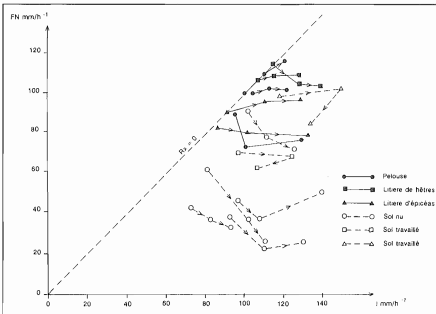
Figure 5 : Relations FN = f(I) pour divers végétations ou états de surface de sols du site du Mont-Lozère (d'après BOUDJEMLINE 1987 ET BOUREGHDA, 1988, simplifié).
