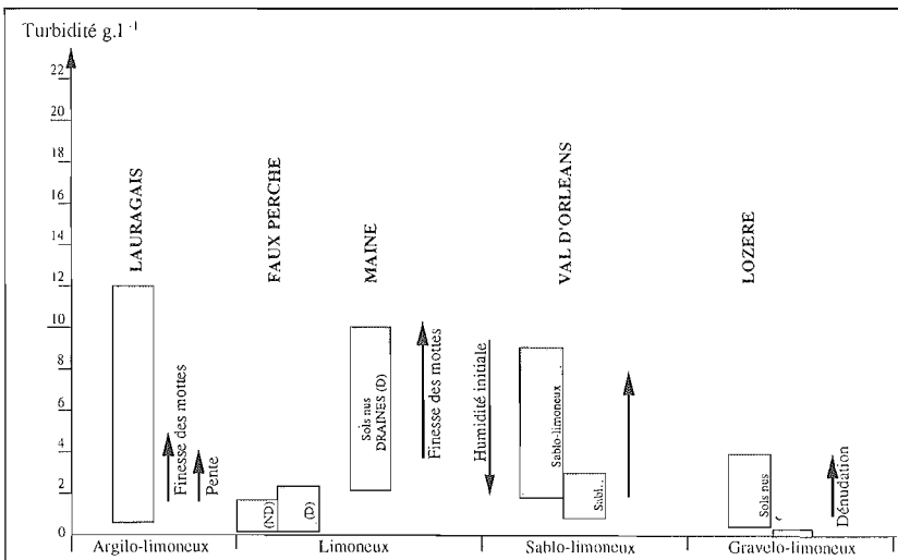
Figure 13 : Plages des valeurs de turbidité (en g.l -1 ) dans les eaux de ruissellement pour les divers types texturaux de sols considérés (pour l = 70 \text{ mm.h}^{-1} ).
