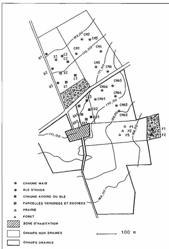
Figure 3 : Plan d'expérience des essais d'aspersion sur le site du Faux-Perche, au lieu dit "La Salmondière" (d'après TRÉVISAN, 1986).
