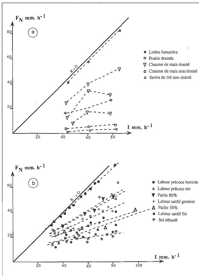
Figure 7 : Relations F_N = f(I) pour différents états de surface des sols du site du Faux-Perche, (a. d'après TRÉVISAN 1986, simplifié) et du Maine (b. d'après RAHELIARISOA, 1986).
