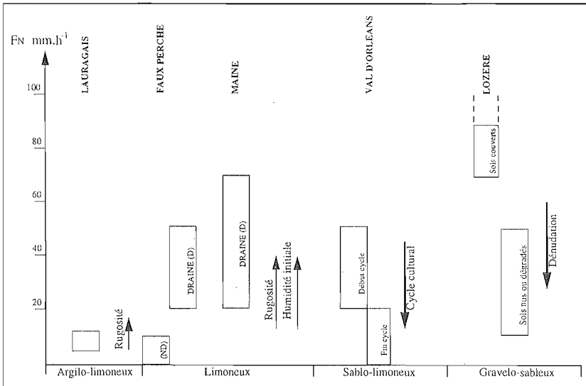
Figure 12 : Plages des valeurs d'infiltrabilité minimales FN (en mm.h -1 ) pour les divers types texturaux de sols considérés (pour l = 70 \text{ mm.h}^{-1} ). NB : les flèches ascendantes (ou descendantes) indiquent l'existence d'une relation positive (ou négative) entre FN et le facteur considéré.
