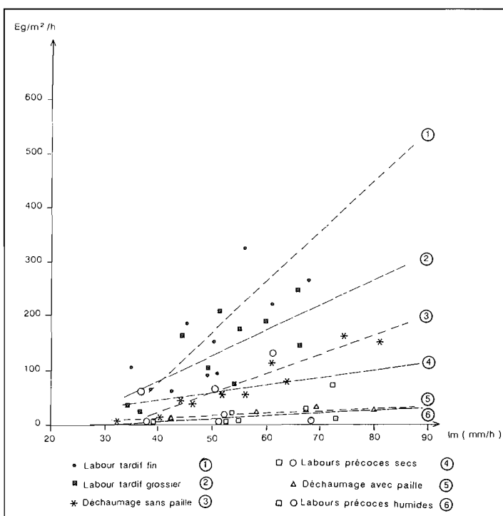
Figure 11 : Variations du débit solide exporté E (en g.m -2 .h -1 ) en fonction de l'intensité des averses pour des parcelles représentatives de six types de lits de semence, sur le site du Maine (d'après RAHELIA-RISOA, 1986). Solid transports versus rainfall intensities for six seed bed types in the site of Maine (from RAHELIA-RISOA, 1986).
