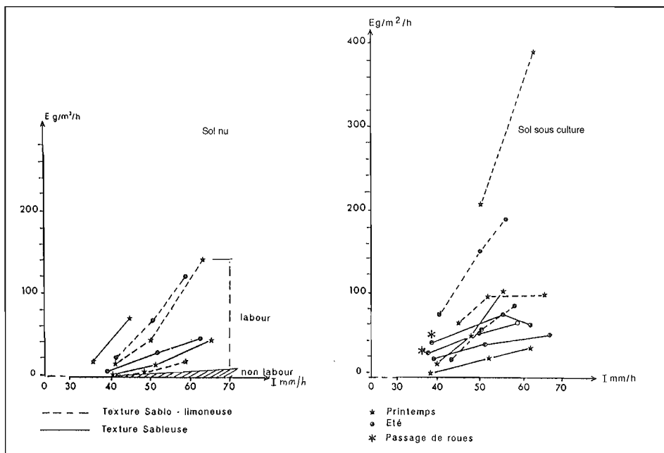
Figure 10 : Variations du débit solide exporté E (en \text{g.m}^{-2}.\text{h}^{-1} ) en fonction de l'intensité des averses I (en \text{mm/h} ) pour deux textures de sol et pour deux stades du cycle cultural, sur le site du Val d'Orléans (d'après RAHELIARISOA)
