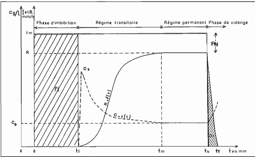
Figure 4 : Hydrogramme théorique de ruissellement R(t) et turbidigramme pour une averse d'intensité constante.
