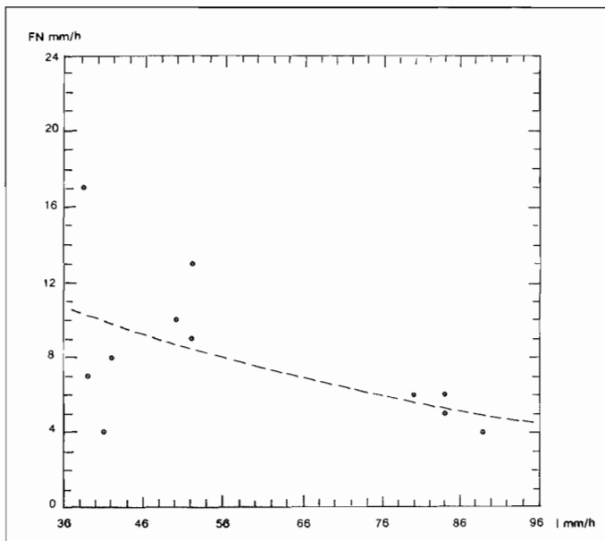
Figure 8 : Relations FN = f(I) , pour 11 parcelles de sol de faible pente (<5%) à surface ratissée, site du Lauragais (d'après BOUDJEMLINE, 1987).
