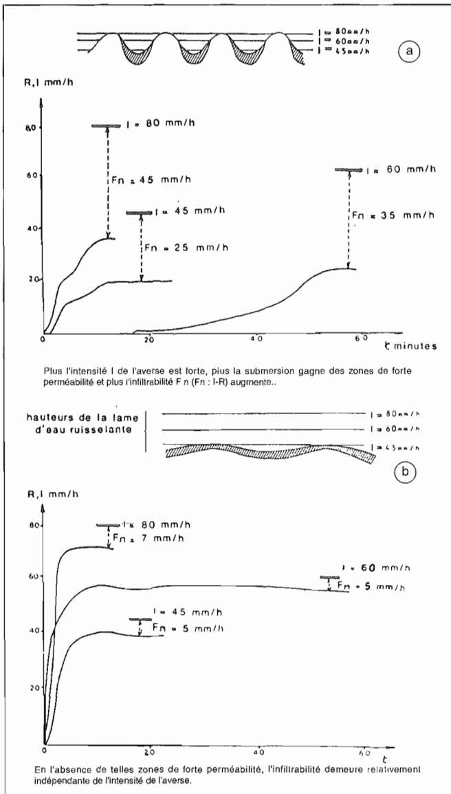
Figure 9 : Hydrogrammes de ruissellement pour 3 intensités d'averses simulées sur 2 parcelles de sol à états de surface contrastés (a) surface rugueuse, (b) surface lisse, homogène. (d'après TREVISAN, 1986).
