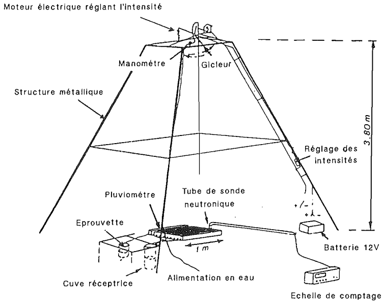
Figure 1 : Vue du dispositif d'aspersion. The rainfall simulation device.
